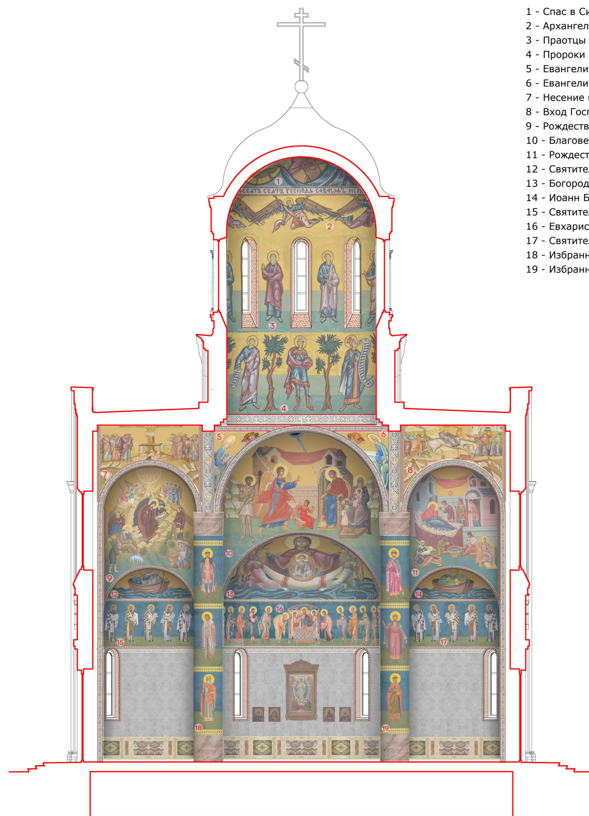
Восточная стена
